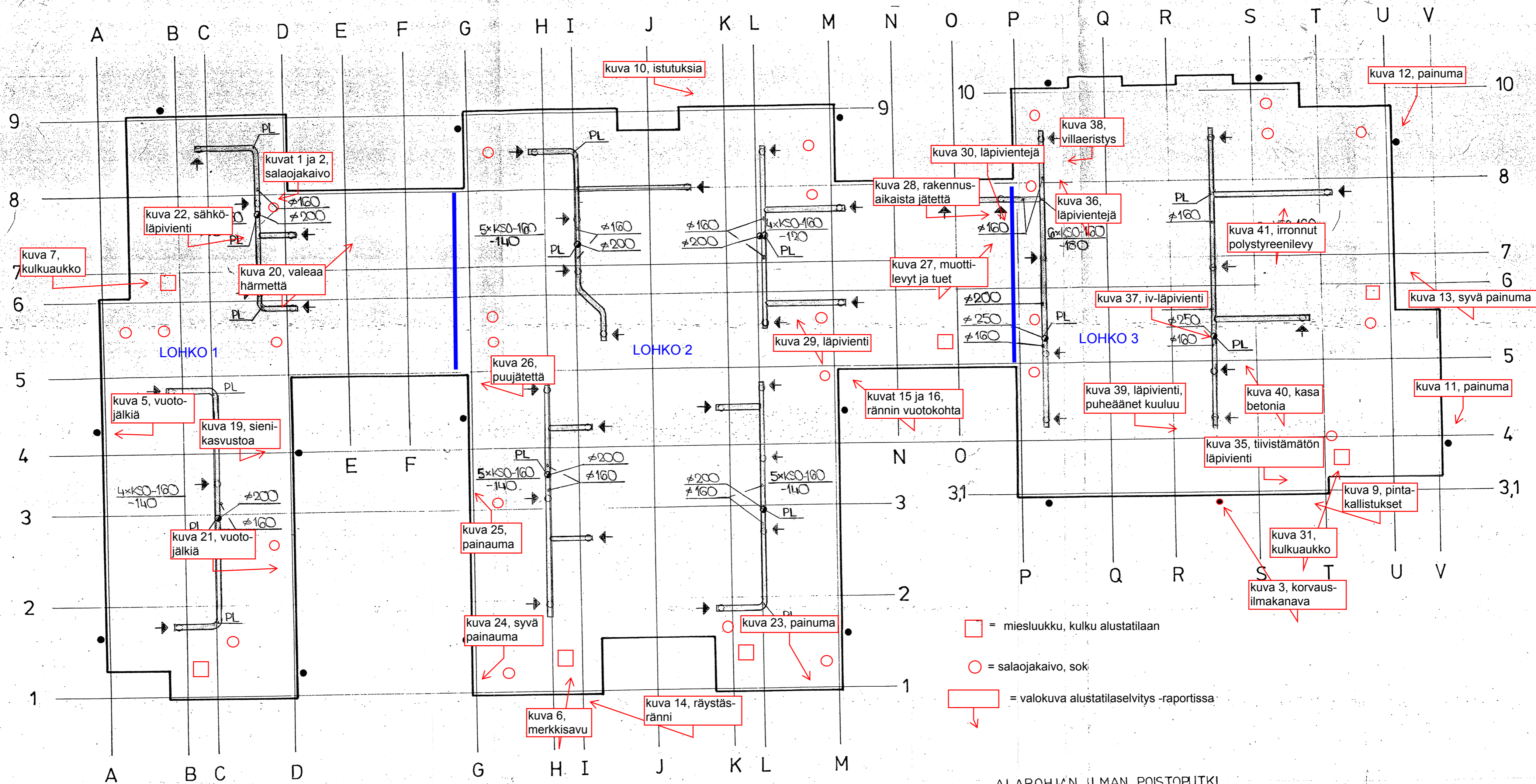
ALAPOHJAN ILMAN POISTOPUTKI MERKITYY ○
