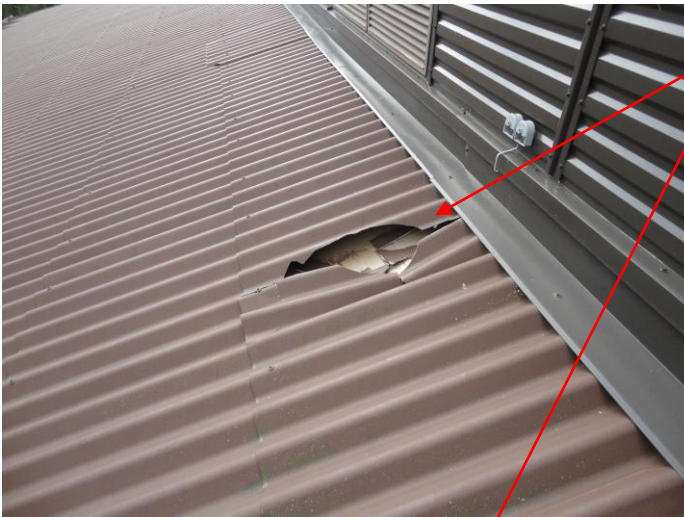
Vesikatteesta lohkeillut paloja irti
